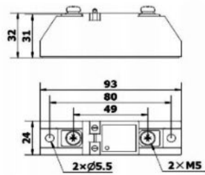
25A-75A尺寸图
