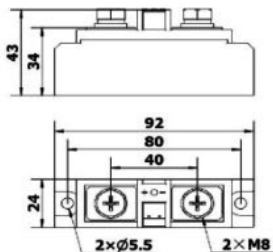
150A-200A尺寸图
