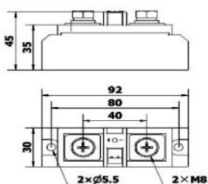
250A-300A尺寸图
