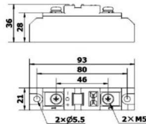
80A-120A尺寸图
