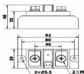
340A-400A尺寸图
